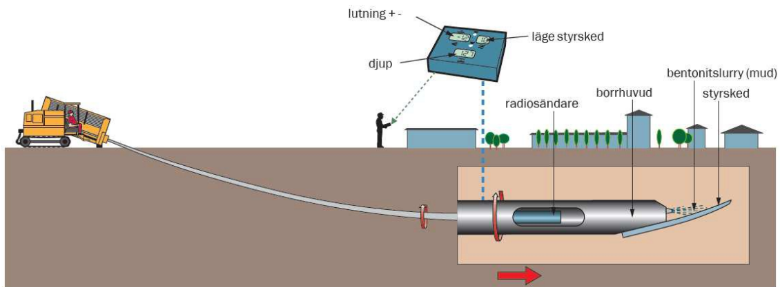
Exempel styrd borrning
