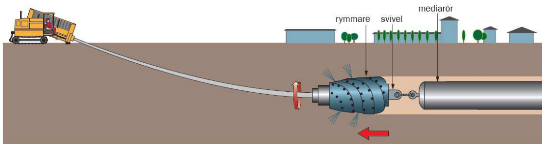
Exempel styrd borring när mediator (kanalisationsrör) dras tillbaka med rymmare.
