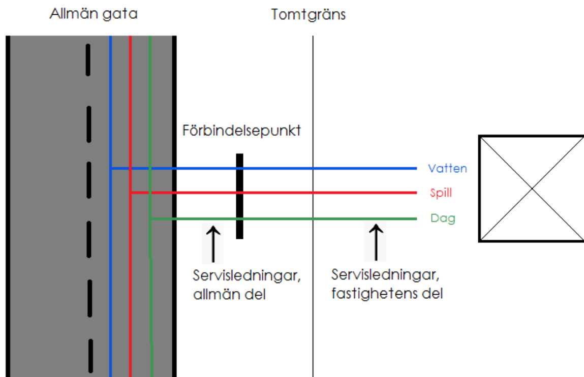
Figur 2. Illustrativ bild över förbindelsepunkten och därmed ansvarsgränsen för VA-huvudman/fastighetsägare.
